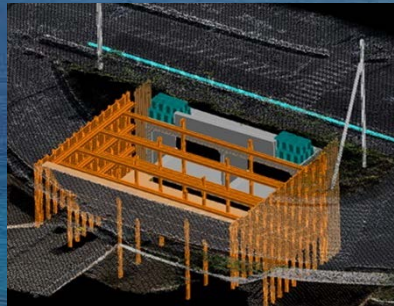
仮設計画
