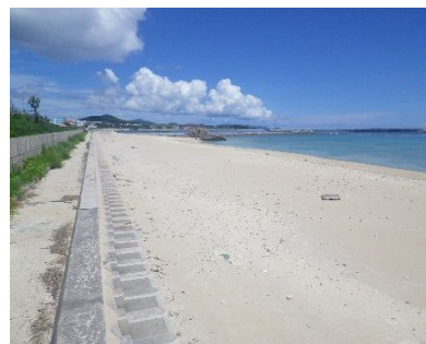
海浜復元・面的防護による高潮対策施設 仲田港（仲田地区）海岸調査測量設計 業務委託（H24）（北部土木事務所）
